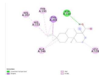
Gambar 17. Visualisasi 2D delta.8(14)-Isopimaric acid dengan Protein 4D0Y
