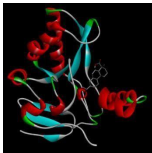
Gambar 16. Abietic acid dengan protein 4D0Y
